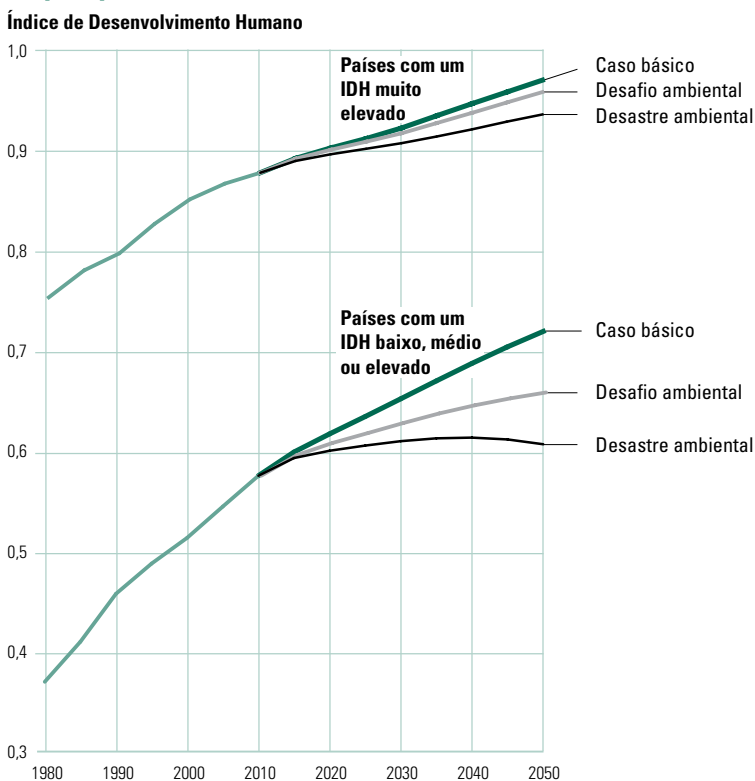
FIGURA 2.5 Cenários que projectam os impactos dos riscos ambientais sobre as perspectivas do desenvolvimento humano até 2050
