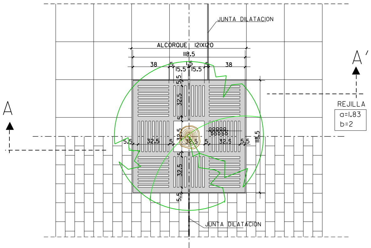
PLANTA E=1:25
