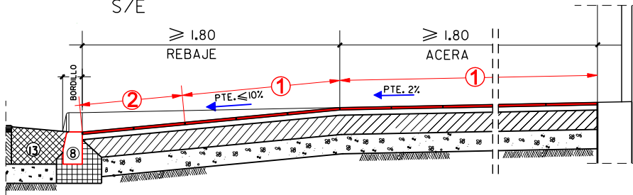
SECCION A-A' S/E
