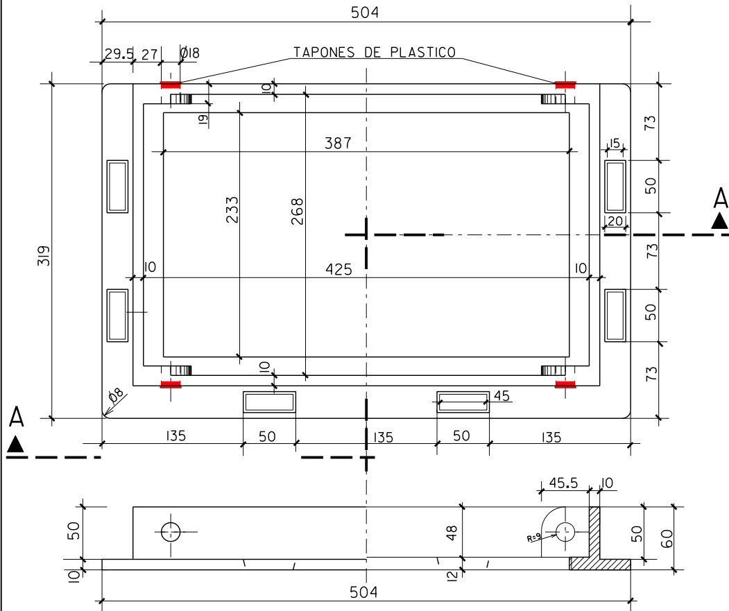
ALZADO-SECCION A-A
