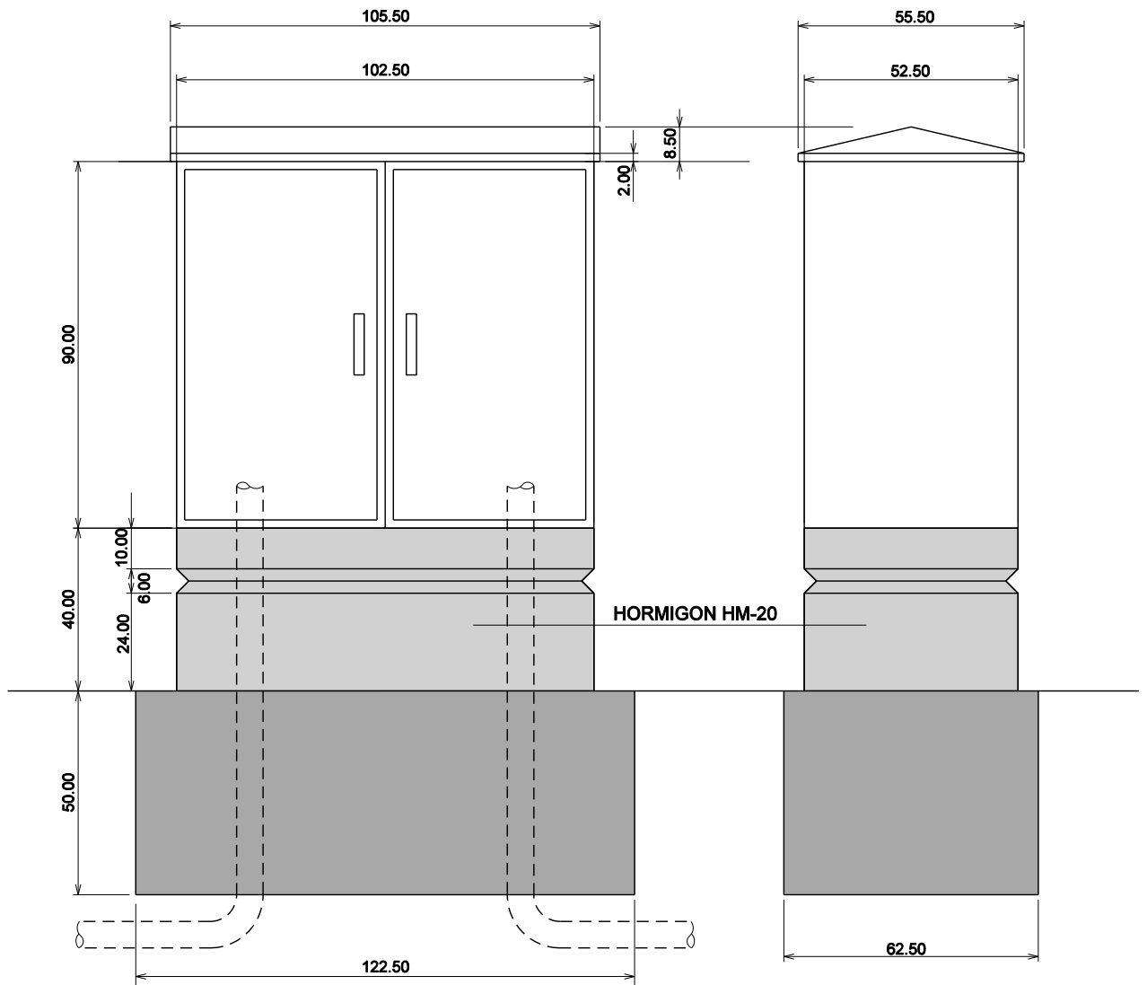
ALZADO
