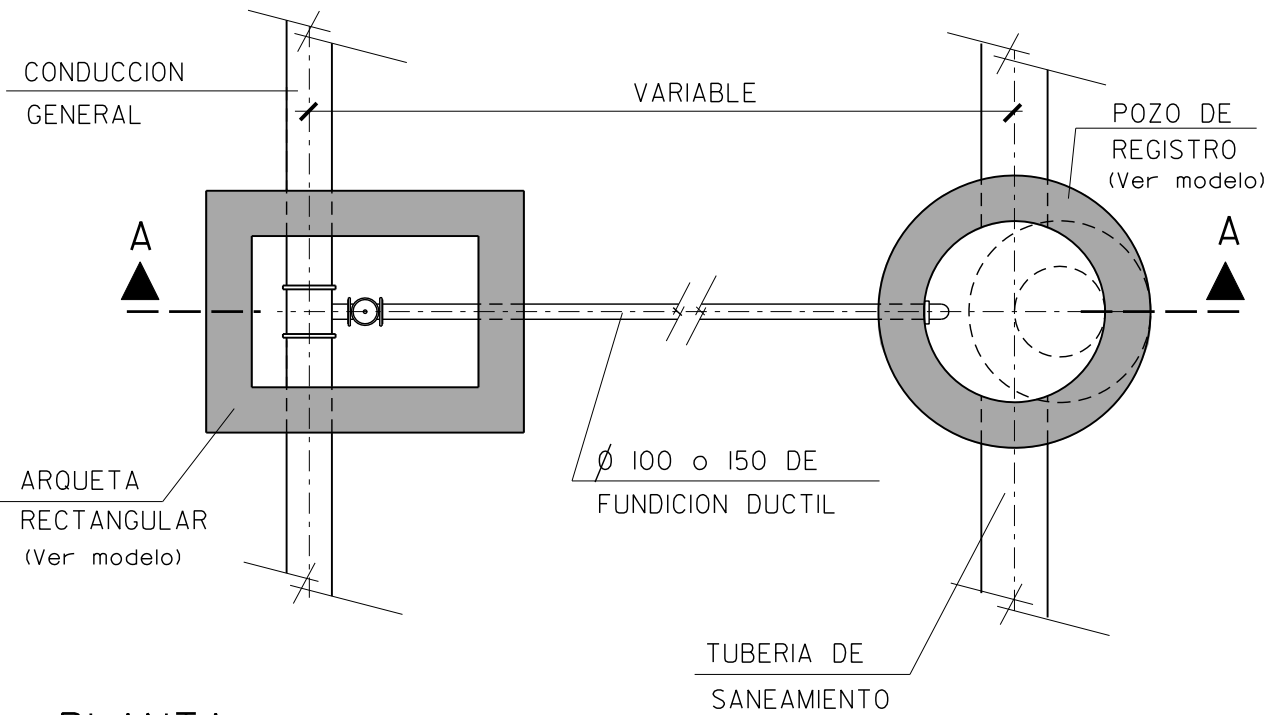
PLANTA
