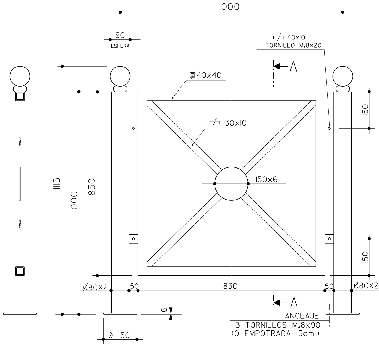
SECCION A-A'
