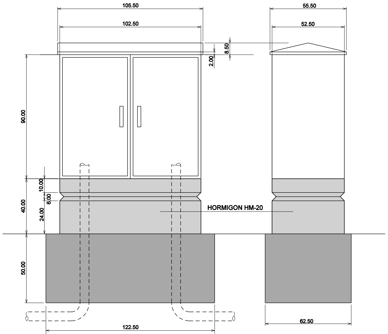
ALZADO
