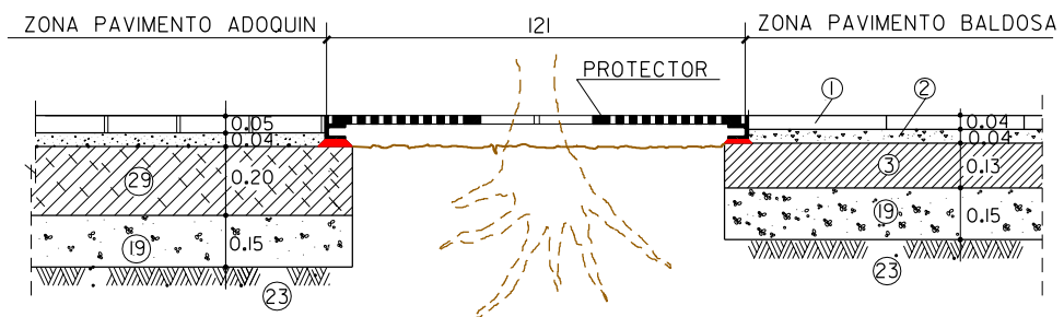
SECCION A-A'
