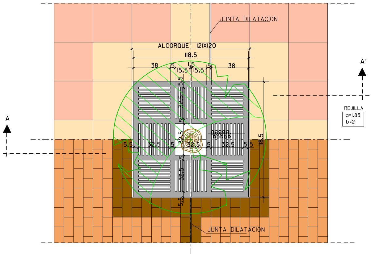
PLANTA
