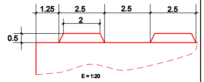
DETALLE BALDOSA ESPECIAL E = 1:20
