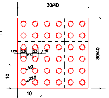
PLANTA E = 1:100
