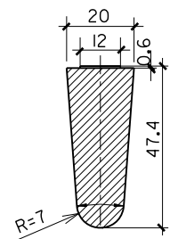
DETALLE NERVIO (a-a) S/E
