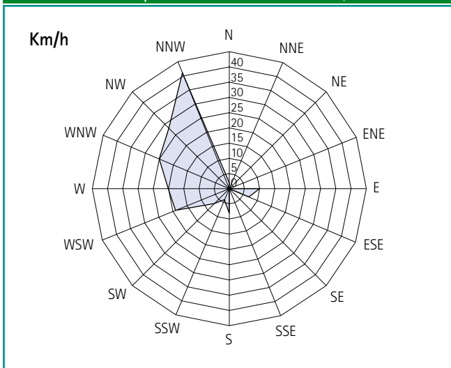
Velocidad media correspondiente al mes de marzo en Km/h en cada rumbo
