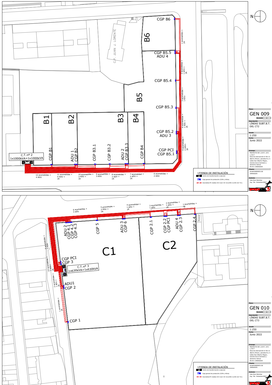
Figura 3: Planos GEN 009 y GEN 010 Planta general Proyecto LSBT
