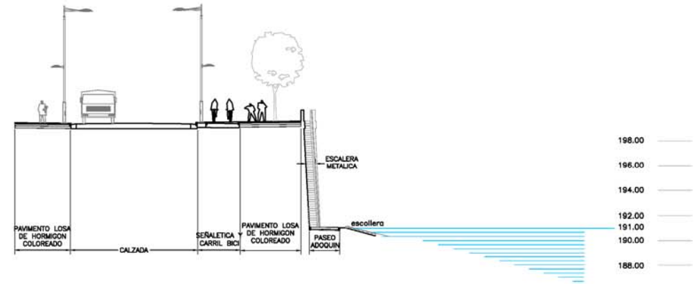
SECCION TRANSVERSAL 1-1
