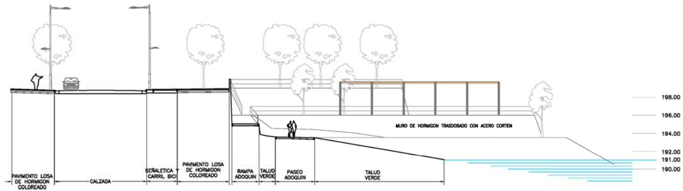
SECCION TRANSVERSAL 2-2
