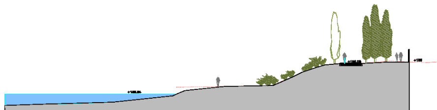
SECCIÓN TRANSVERSAL ①
