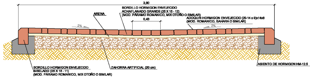
DETALLES DE PAVIMENTOS CAMINO PERIMETRAL 1 Y 3 E:1/20
