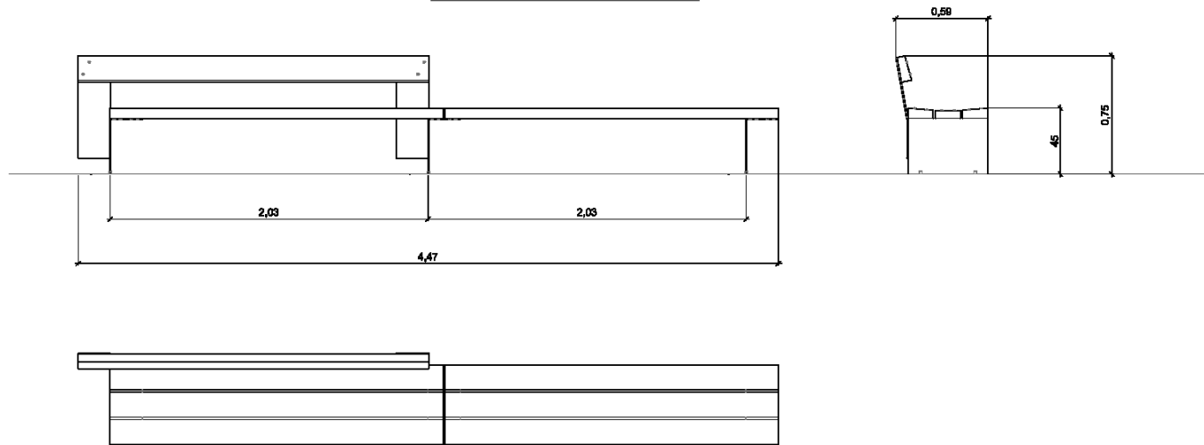
DOS TRAMOS CON UN RESPALDO. TIPO 3
