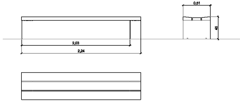
UN TRAMO SIN RESPALDO. TIPO 1
