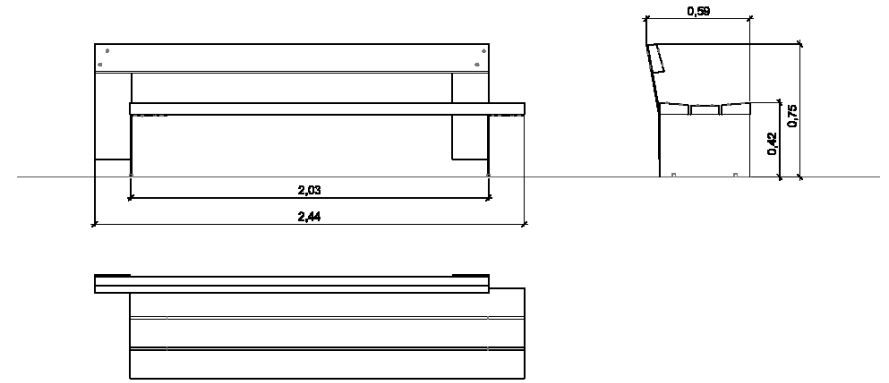
UN TRAMO CON RESPALDO. TIPO 2
